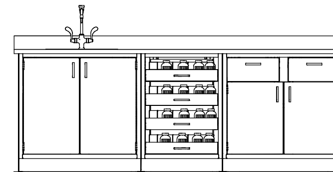
Elevation E
